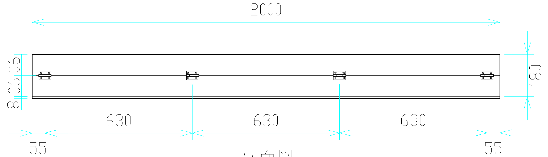
立面図 〈場外側〉
