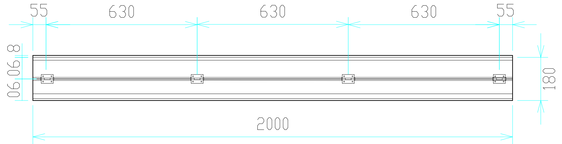
立面図 〈現場側〉
