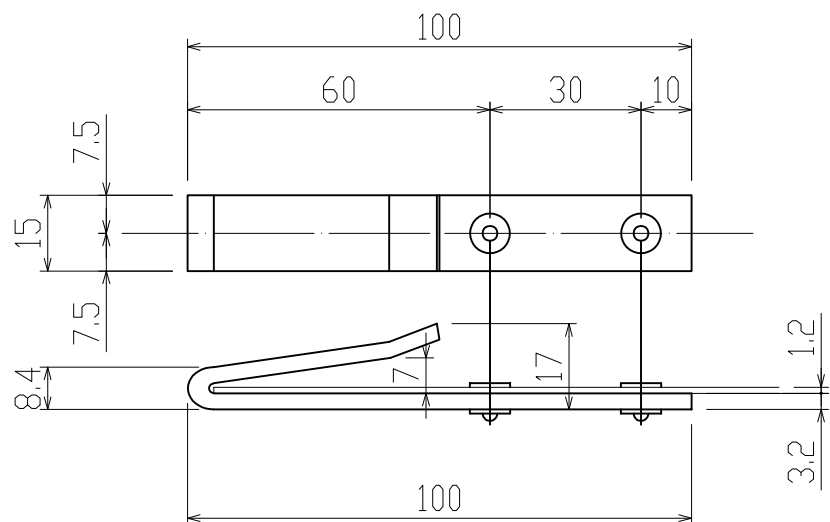
引っ掛けフック詳細図 1/1.5
