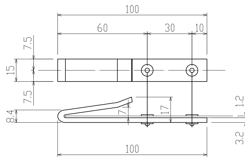
引っ掛けフック詳細図 1/1.5
