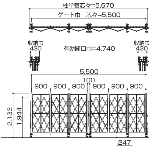
サイクルカスターゲート (CCGA-2027 + CCGA-2027)
