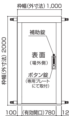
立面図（ドアパネル部・表）
