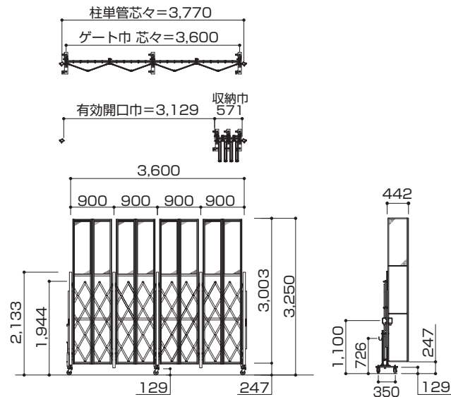
サイクルカスターゲート (CCGA-3036)
