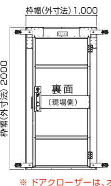
立面図（ドアパネル部・裏）
