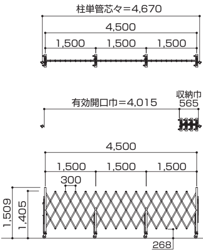
サイクルクロスゲート（CXGA-1545）
