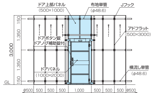
立面図（現場側・h3000mm仕様）
