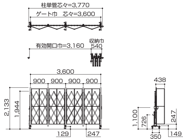
サイクルカスターゲート (CCGA-2036)
