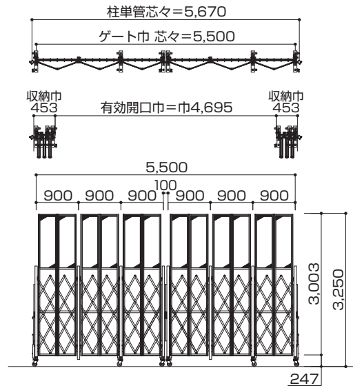
サイクルカスターゲート (CCGA-3027 + CCGA-3027)
