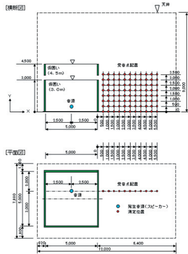
<図1:音源、受音点、仮囲い壁の配置>
