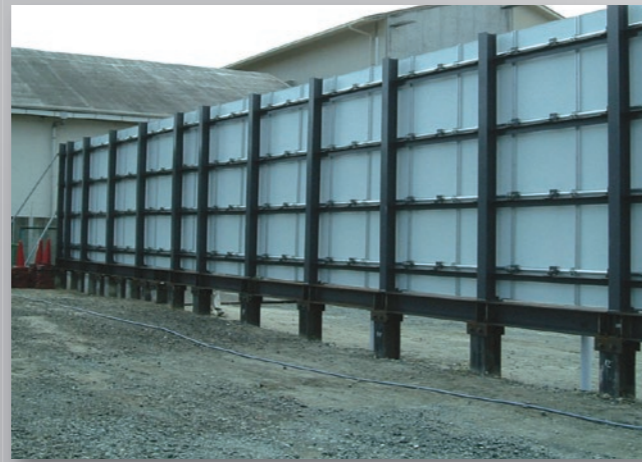
鉄道沿線工事物件 周辺住民 防音対策と美観性・強度(H:3000mm仕様)
