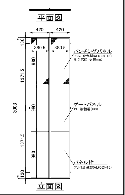
【パネル部分詳細図】
