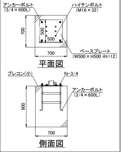
【パネル部分詳細図】
