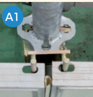
コーナー以外の干渉する直線部に取付けた例
