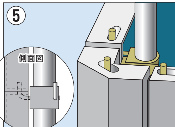
防音パネルを下から出ているクランプフックにクランプ孔を通す。
