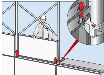
パネルをクランプから外す。 ※メバリにテープ等を使用した場合は、 テープ等を取り除いてからパネルを 外す。
