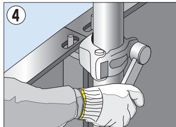
クランプ金具のネジをしっかりと締める。
