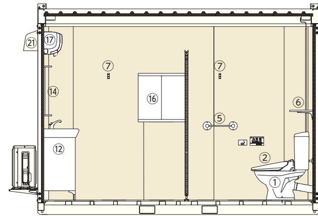
正面図
