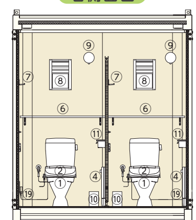
右側面図
