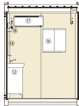
右側面図
