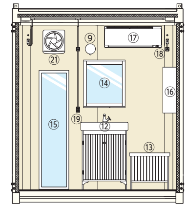
左側面図
