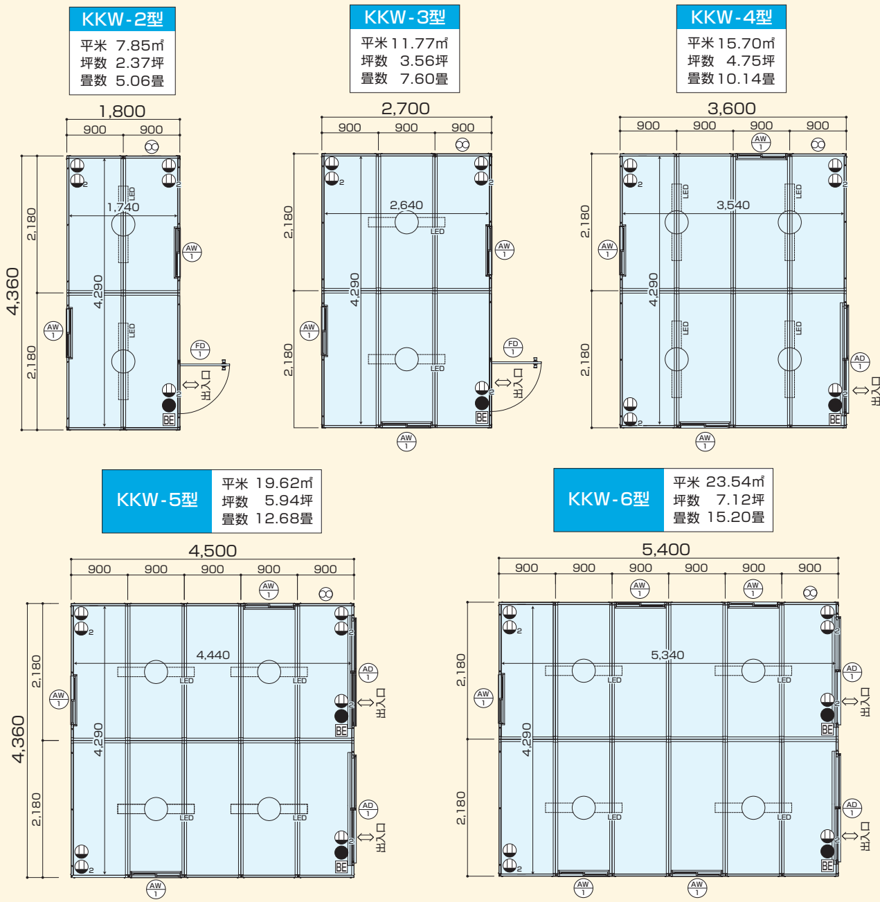
■ 平面図 (妻2連棟 桁2連棟～桁6連棟)
