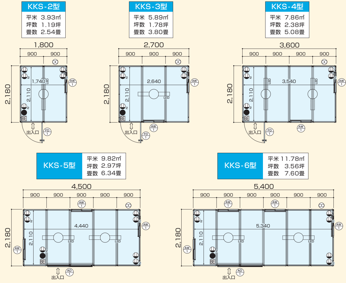
■ 平面図 (桁2連棟～桁6連棟)
