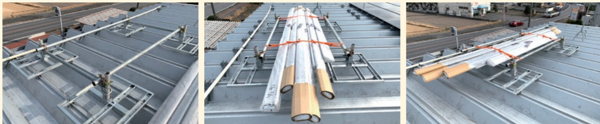
荷受け架台を屋根上に設置できるので、部材等を安定させたまま、養生・保管が行えます。
