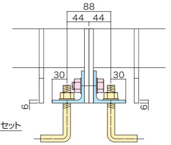
■ 設置図 (連棟部)
