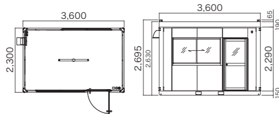
■ TM-36型
