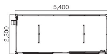
■ TM-54型
