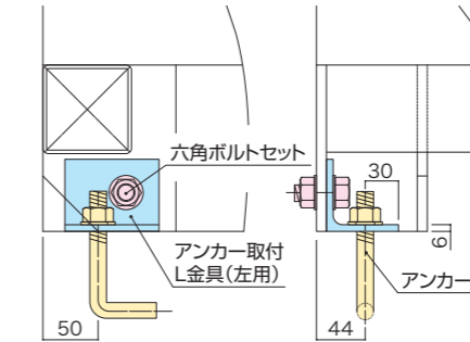
■ 単棟部アンカー取付イメージ
