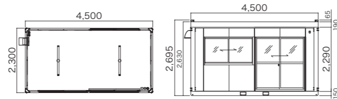
■ TM-45型
