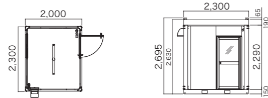
■ TM-20型
