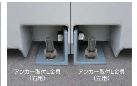
■ 連棟部アンカー取付イメージ
