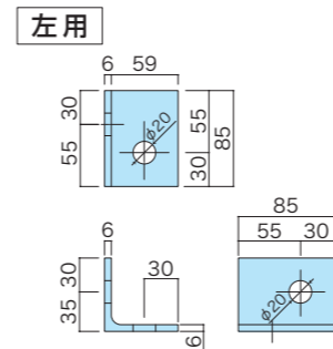
■ アンカー取付L金具寸法図
