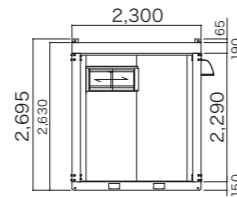
■ TM-45型
