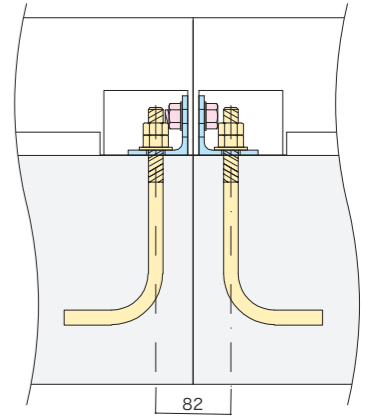
■ 連棟部アンカー取付イメージ
