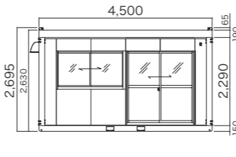
■ 妻側立面
