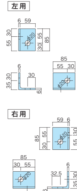
■ アンカー取付L金具寸法図
