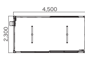
■ TM-45型
