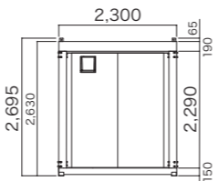
■ 妻側立面
