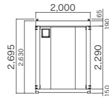
■ 妻側立面
