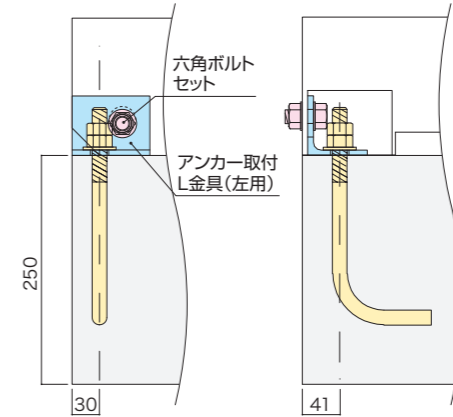
■ 単棟部アンカー取付イメージ
