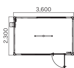
■ TM-36型
