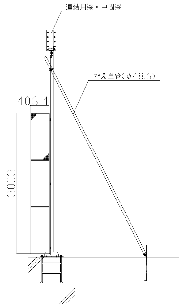
側面図
