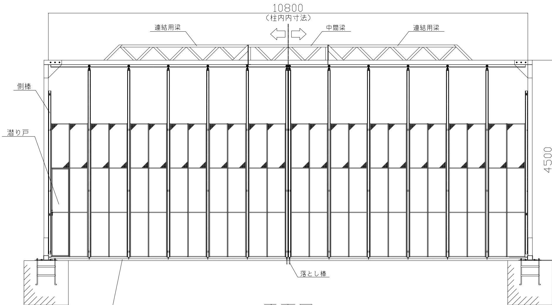
正面図
