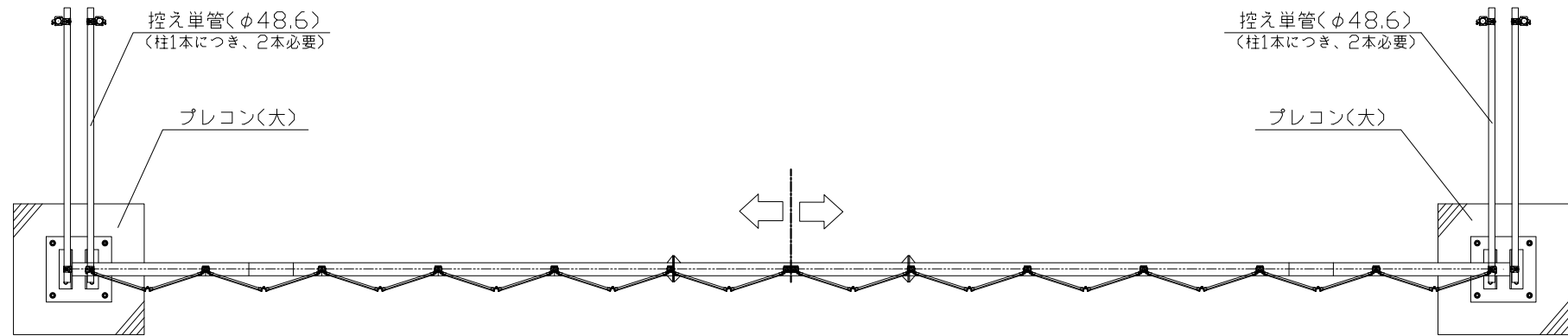
平面図
