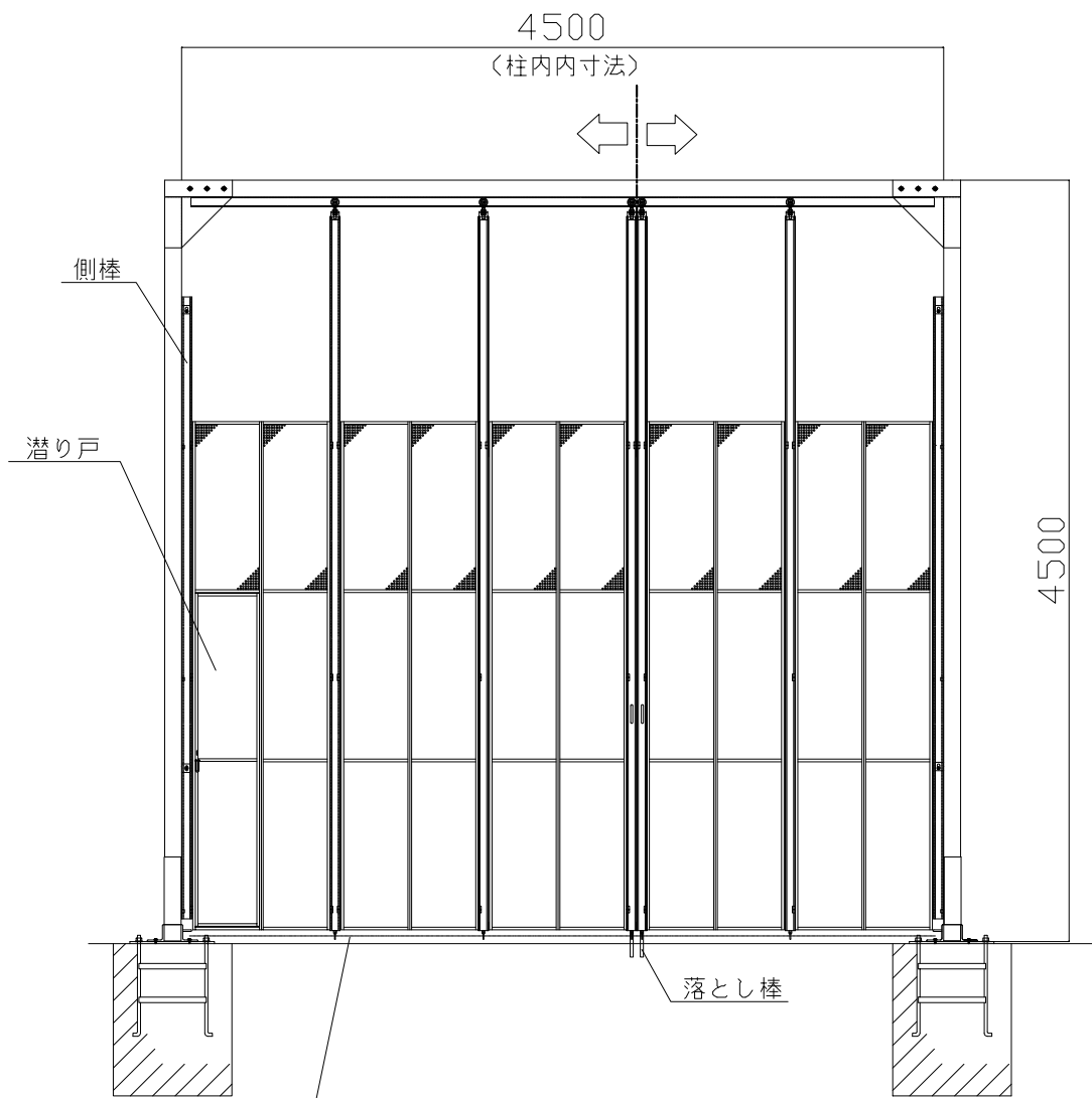
正面図
