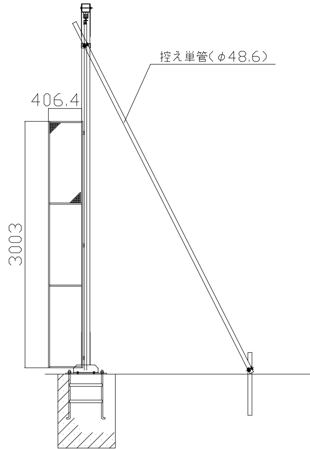
側面図
