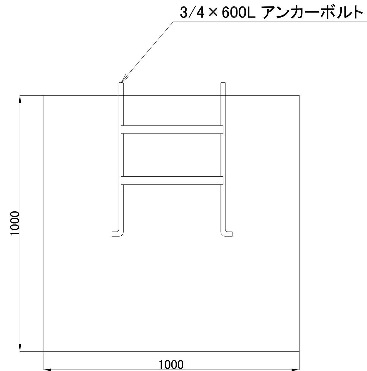
側面図
