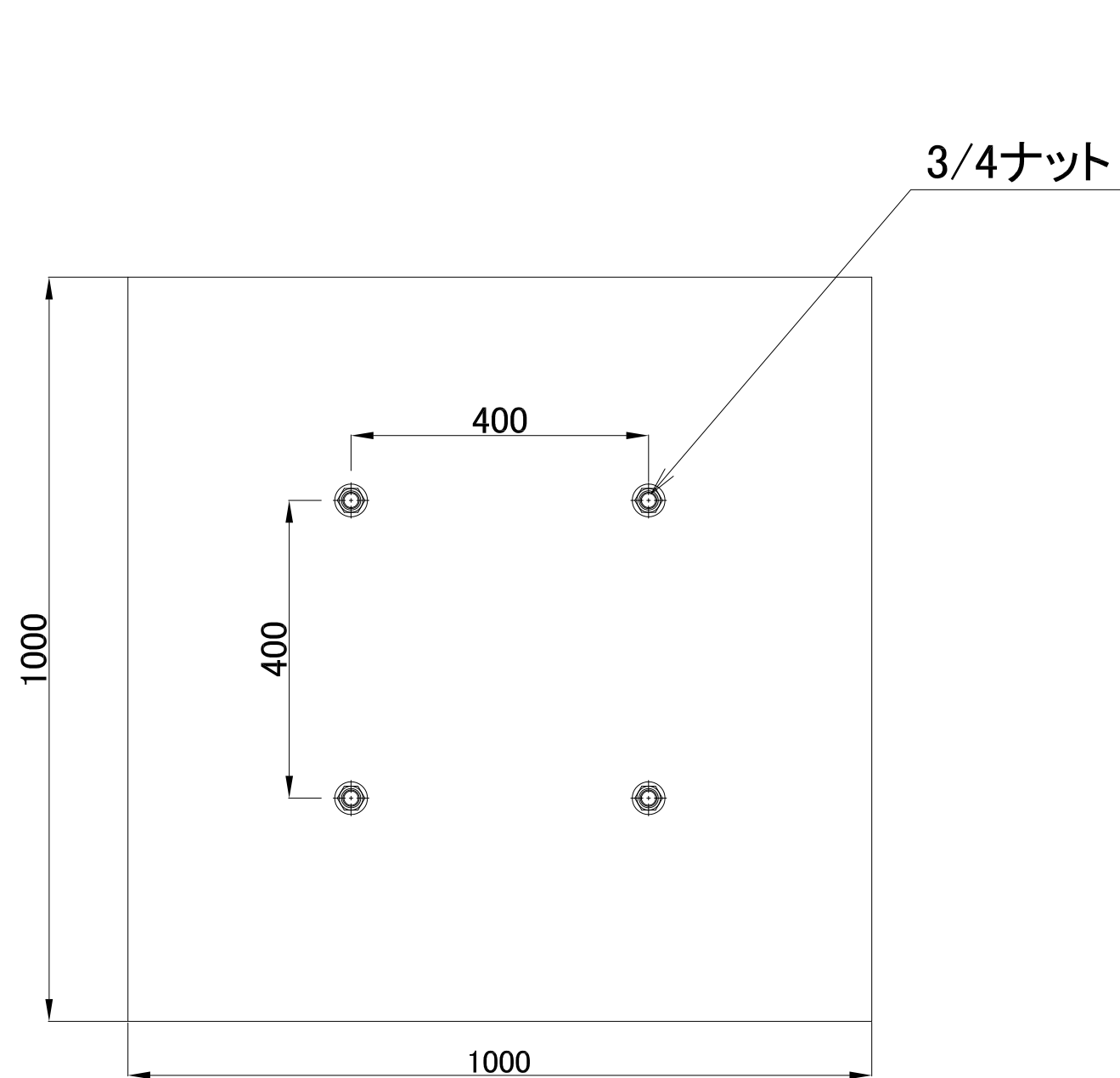
平面図
