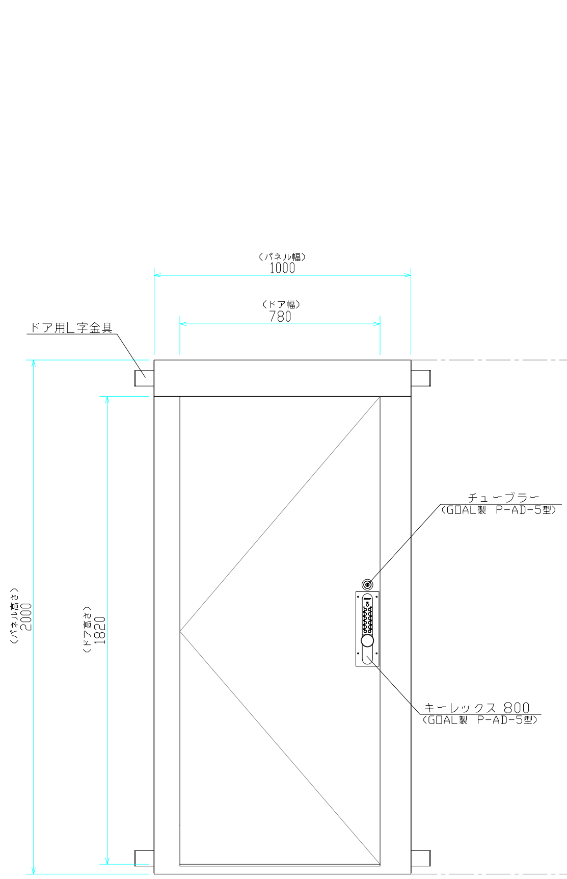
立面図 (場外側)
