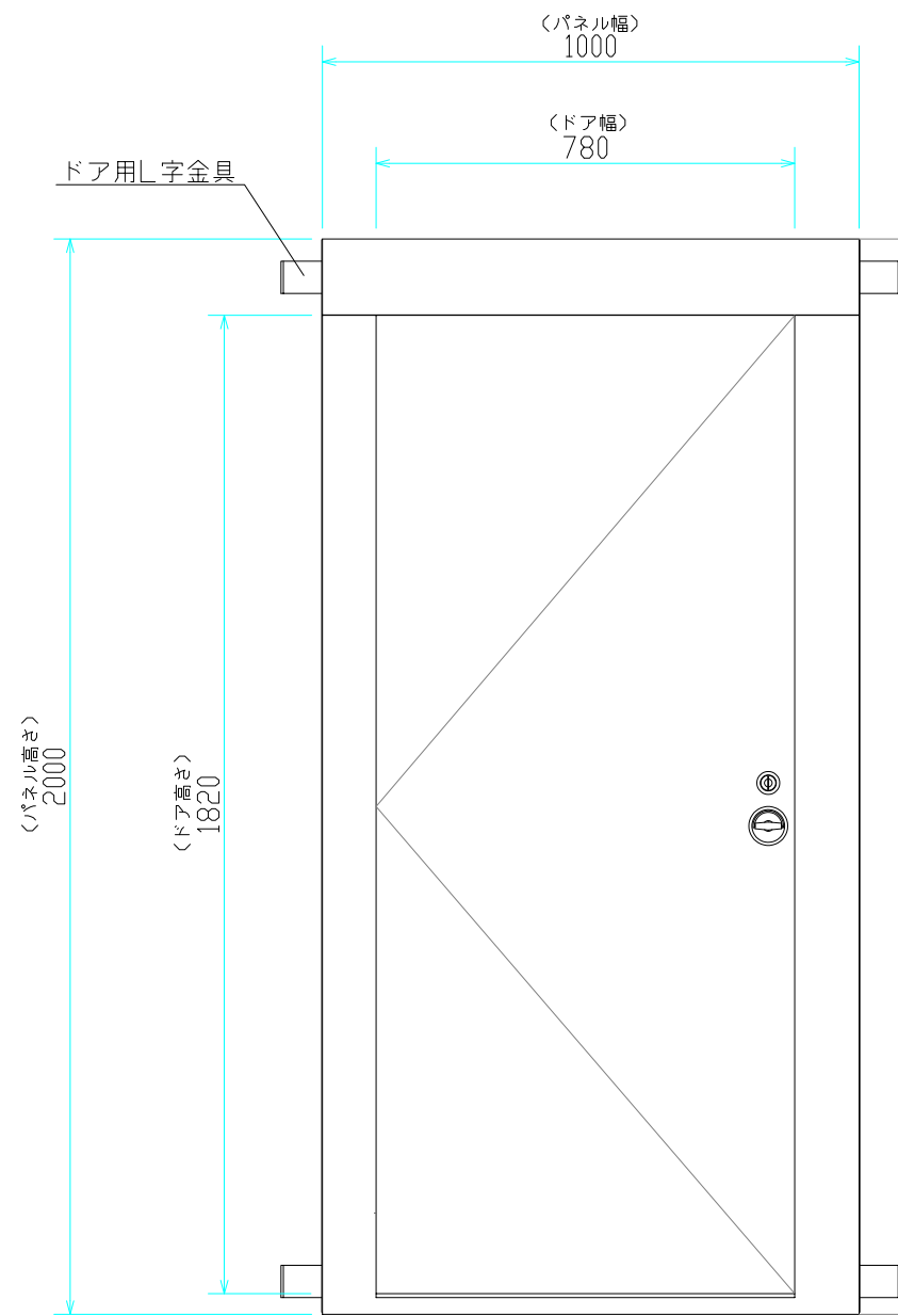
立面図 (場外側)
