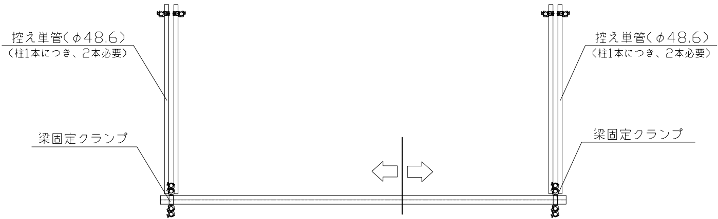
平面図
