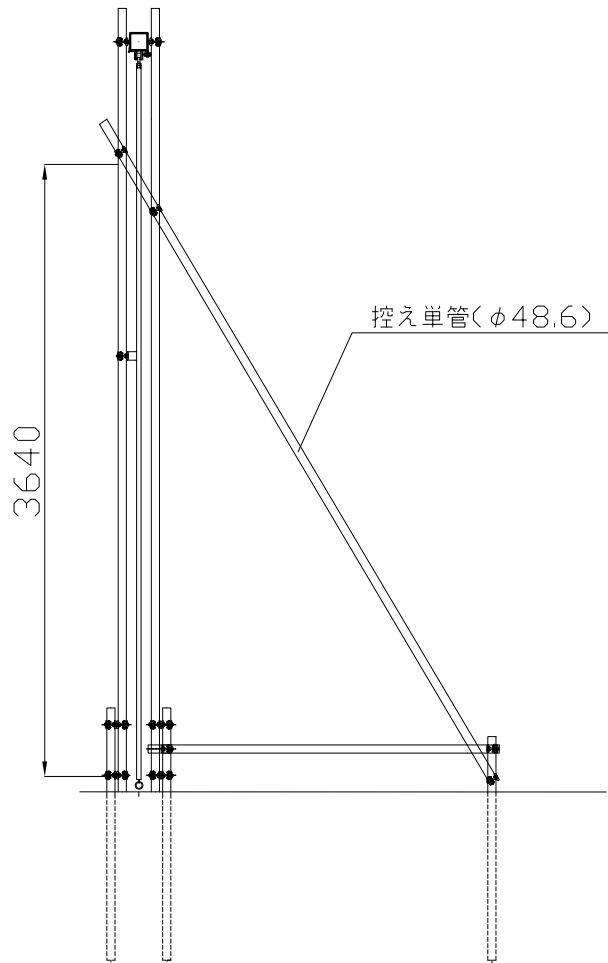
側面図
