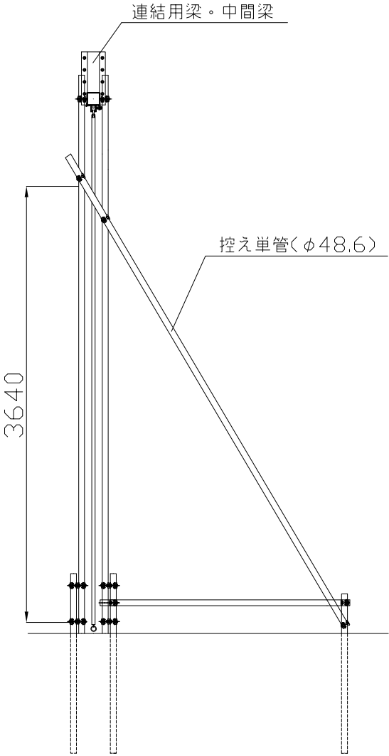
側面図
